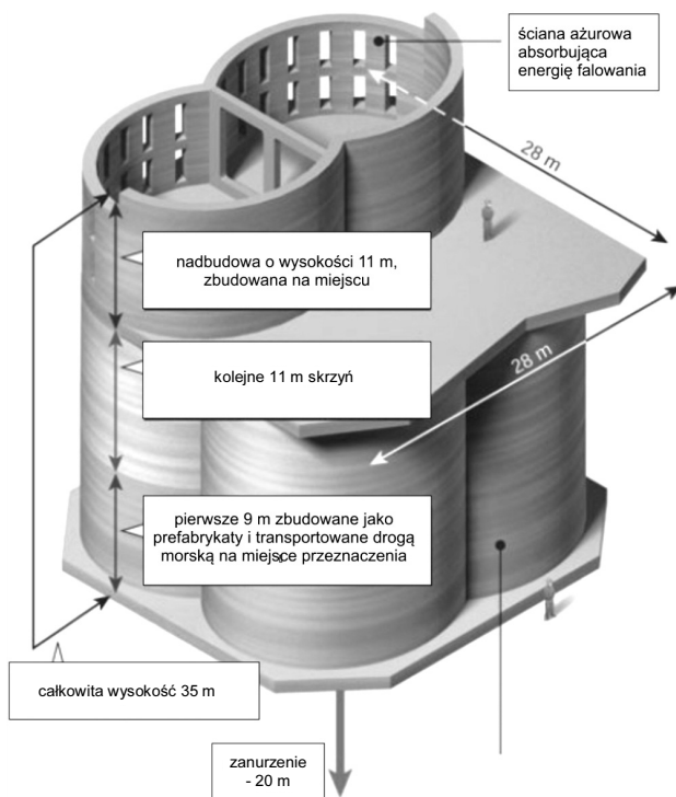
Rys. 6. Rysunek poglądowy czterekomorowej konstrukcji skrzyni, Tanger (Maroko)
