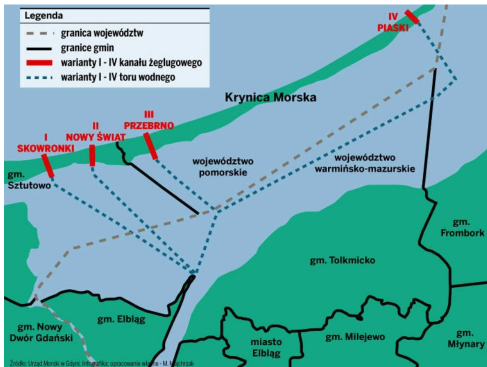
Rys. 3. Propozycje miejsc budowy kanału żeglownego w poprzek Mierzei Wiślanej
