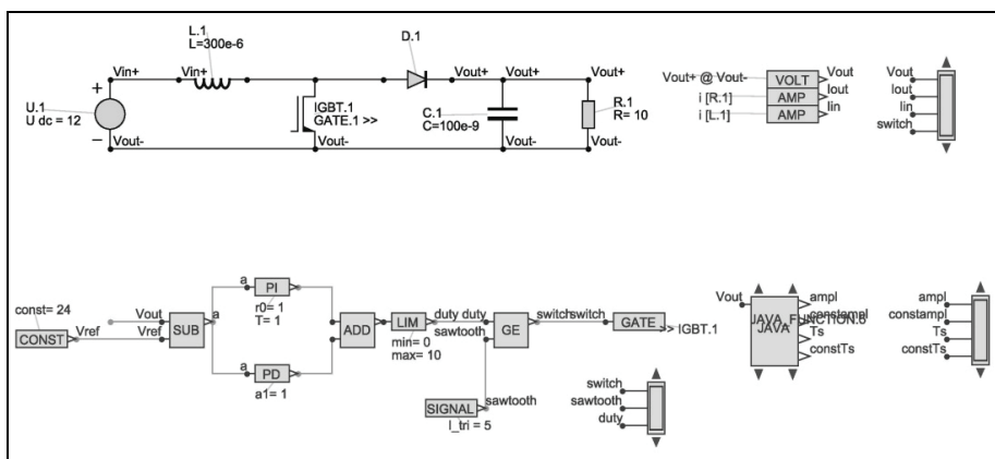
Rys. 2. Układ przekształtnika boost zaprezentowany w środowisku GeckoCIRCUITS
